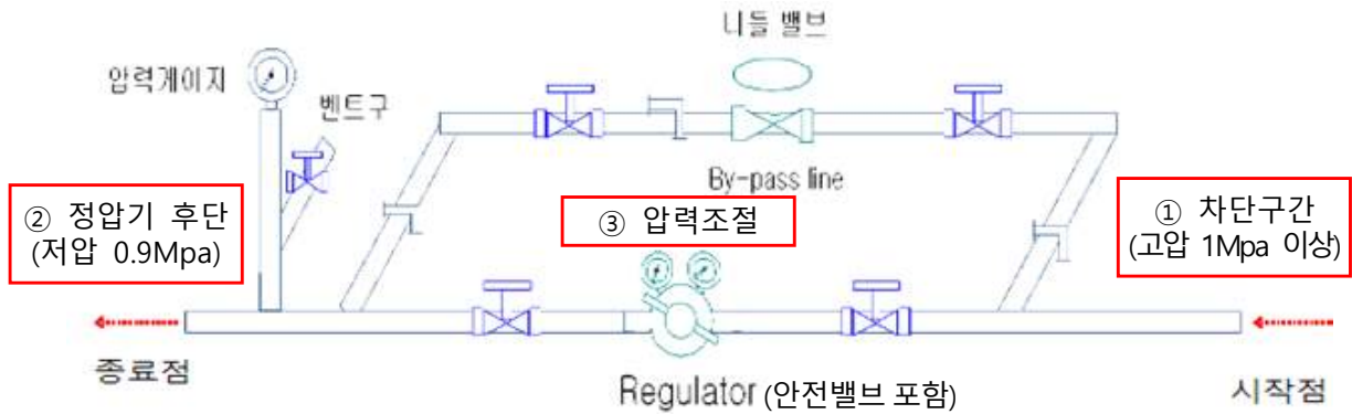
【그림】 고압가스회수장비 설비구조 도면
